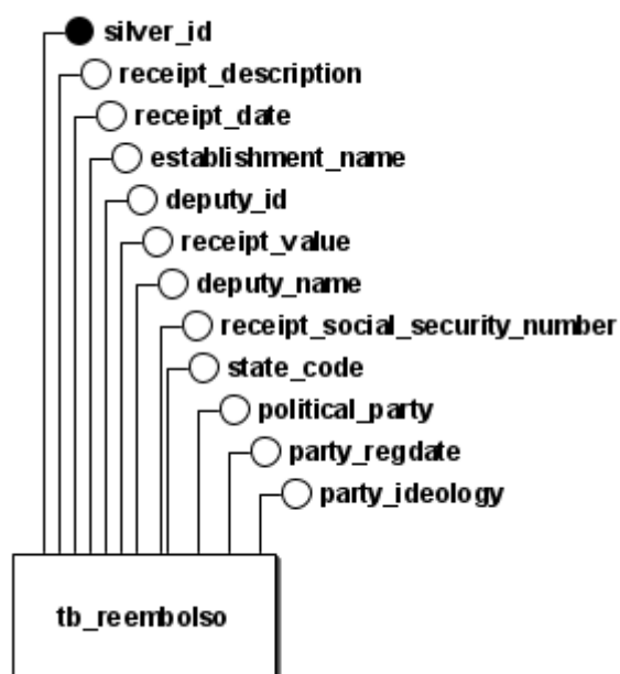
Figura 1 – Diagrama Entidade-Relacionamento (DER) da camada Silver
